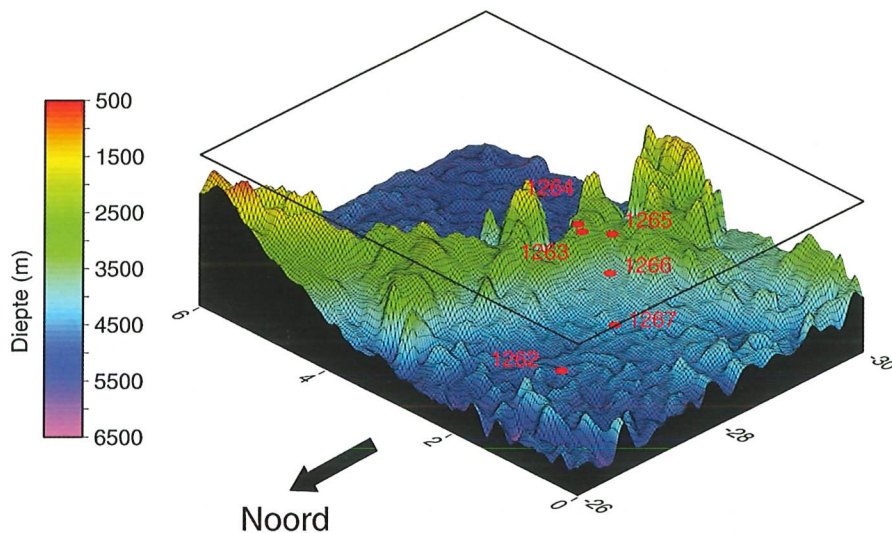
Figuur 7. Een drie-dimensionaal beeld van de topografie van de oceaanbodem (bathymetrie) van de Walvis Ridge voor de zuidwestkust van Zuid-Afrika. De rode stippen met nummers geven de positie van de boringen weer. Het zwarte vierkant geeft het oceaanooppervlak aan.
