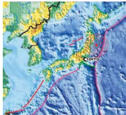
Afb. 1. De Tohoku-beving vond plaats op 24 kilometer diepte onder de zeebodem. Bron: USGS
