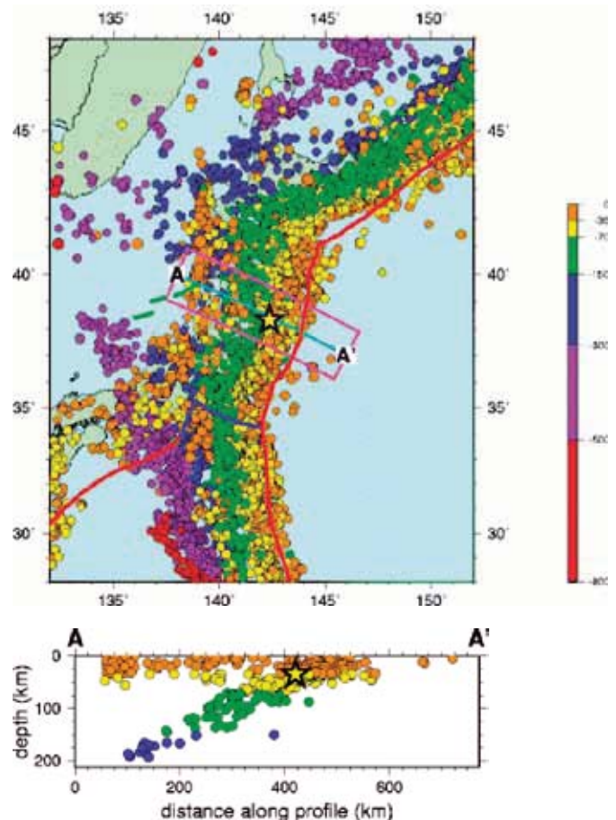
Afb. 4. (A en B) Doorsnede door Japan langs de profiellijn in de bovenste figuur. De registratie van de (diepte van de) aardbevingen geeft een duidelijk beeld van de neerduikende plaat (onder). Bron: USGS
